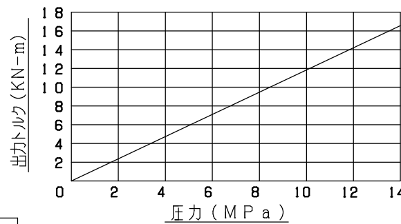
出力(トルク)性能表
