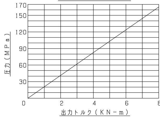
出力(トルク)性能表
