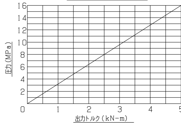
出力(トルク)性能表
