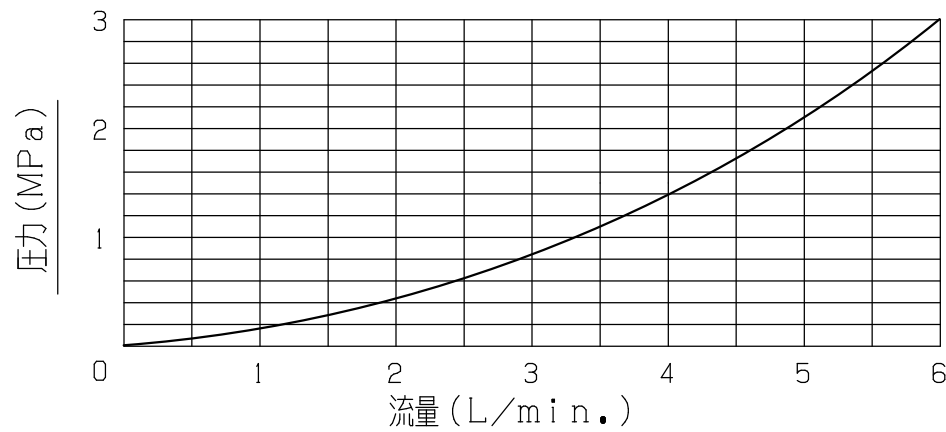
圧力降下特性 (弁全開時)
