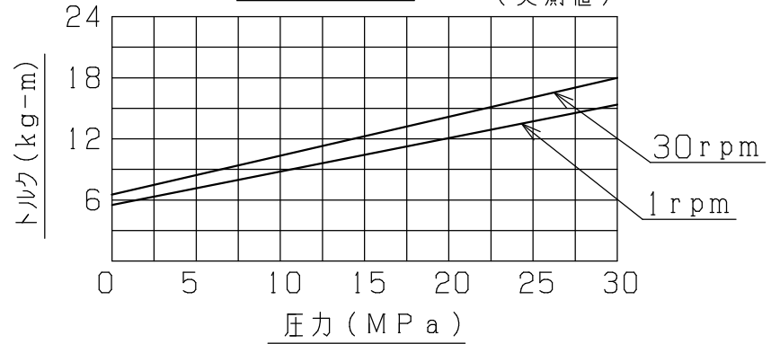
トルク性能表 (実測値)
